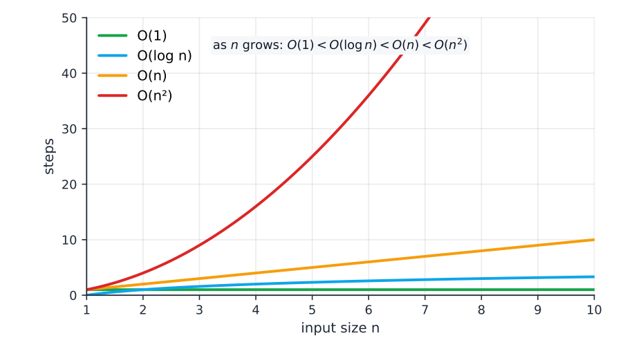
常见复杂度下, 步数随输入规模增长的情况
