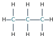
Propane · C_3H_8
