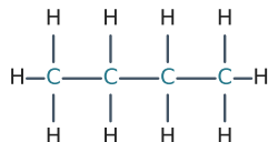
Butane · C_4H_{10}
