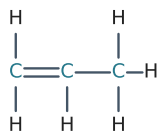
Pentene · C 5 H 10
