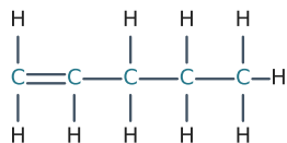
Pentene · C 5 H 10
