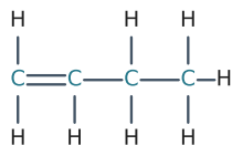
Butene · C 4 H 8
